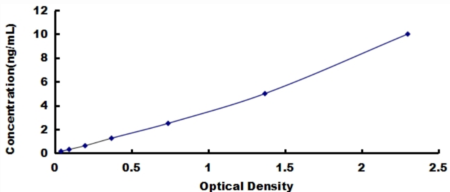
Typical Standard Curve of ELISA Assay for Human, KL.
