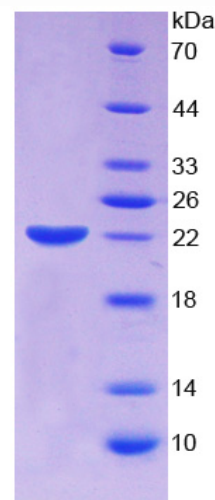
15% SDS-PAGE
